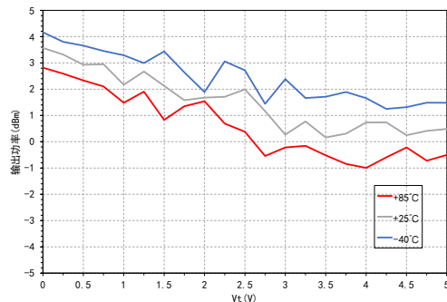
RF/8输出功率VS调谐电压
