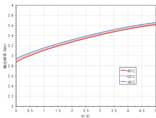
RF/8输出频率VS调谐电压
