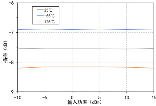
中心频点插损VS输入功率@Vt=12V
