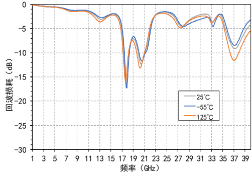
输出回波损耗VS频率@Vt=12V
