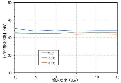
1/2F0带外抑制VS输入功率@Vt=12V
