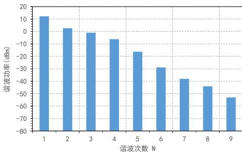
谐波功率 VS 谐波 (Pin=18dBm,Fin=5GHz)
