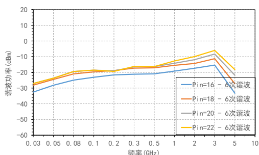
谐波功率 VS 频率
