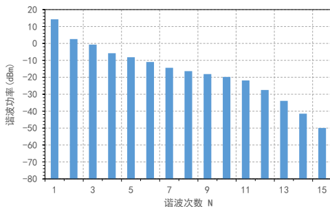
谐波功率 VS 谐波 (Pin=20dBm,Fin=2GHz)
