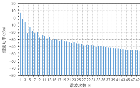
谐波功率 VS 谐波 (Pin=20dBm,Fin=0.2GHz)
