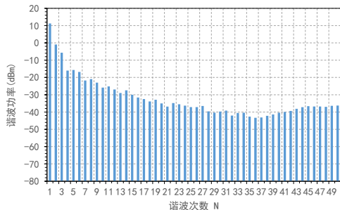
谐波功率 VS 谐波 (Pin=18dBm,Fin=0.5GHz)
