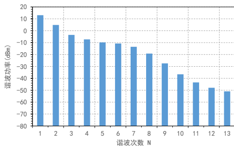
谐波功率 VS 谐波 (Pin=18dBm,Fin=3GHz)
