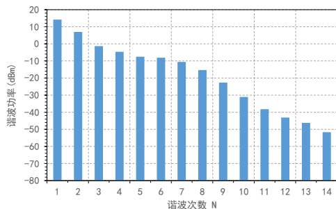
谐波功率 VS 谐波 (Pin=20dBm,Fin=3GHz)
