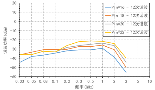
谐波功率 VS 频率
