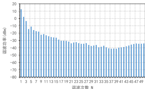
谐波功率 VS 谐波 (Pin=20dBm,Fin=0.5GHz)
