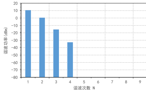
谐波功率 VS 谐波 (Pin=20dBm,Fin=10GHz)
