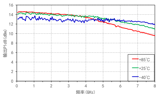
输出P1dB VS 频率@温度
