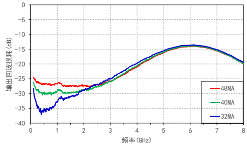
输出回波损耗 VS 频率@电流
