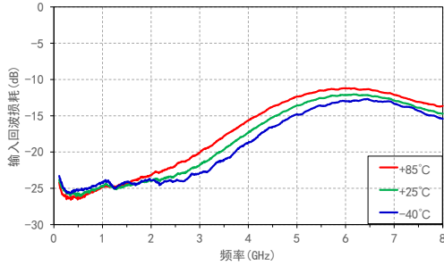
输入回波损耗 VS 频率@温度
