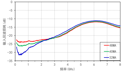
输入回波损耗 VS 频率@电流
