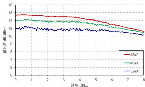
输出P1dB VS 频率@电流
