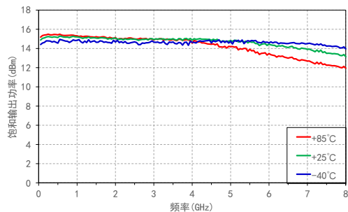
饱和输出功率 VS 频率@温度
