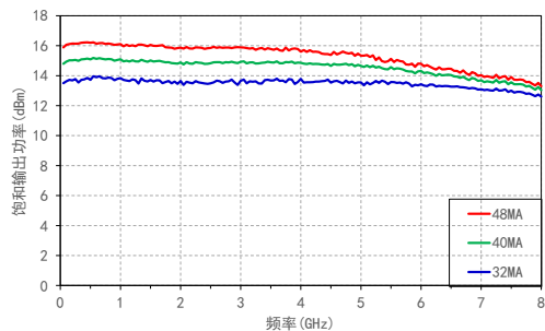
饱和输出功率 VS 频率@电流
