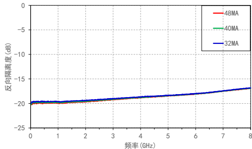
反向隔离度 VS 频率@电流
