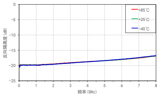
反向隔离度 VS 频率@温度
