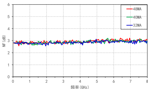
噪声系数VS 频率@电流
