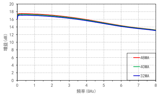
增益 VS 频率@电流
