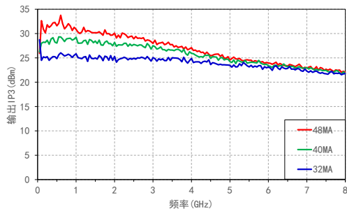
输出IP3 VS 频率@电流
