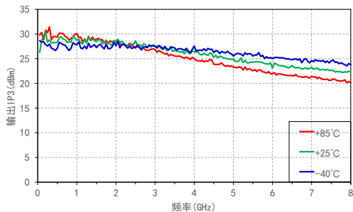
输出IP3 VS 频率@温度
