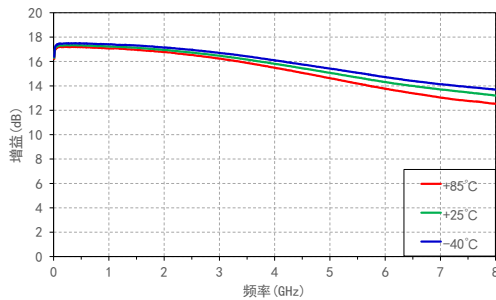
增益 VS 频率@温度
