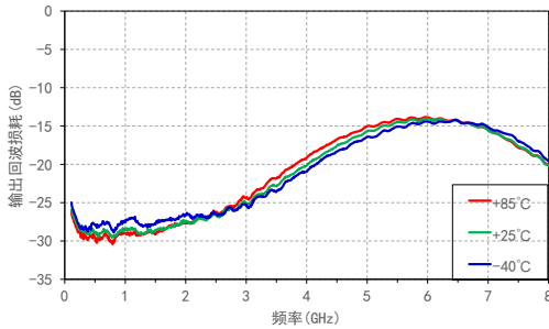
输出回波损耗 VS 频率@温度
