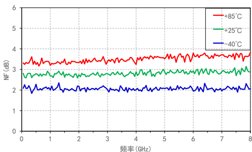
噪声系数 VS 频率@温度
