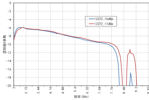
变频增益VS频率
