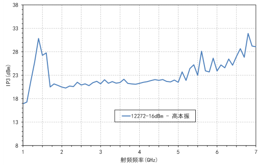
IP3 VS 射频频率(高本振)
