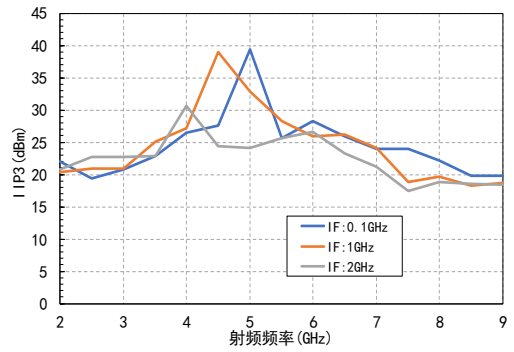
IIP3 VS 射频频率 (高本振)
