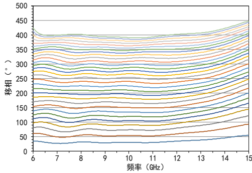
移相VS频率@Pin=-10dBm (Vt=0.5V~15V)
