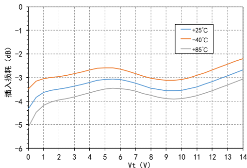
插入损耗VS Vt@=10GHz
