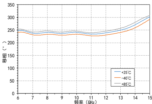
移相VS频率@Vt=7V
